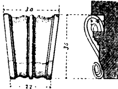
Fig. 12ª Sorraglia degli archi del 2° piano.
