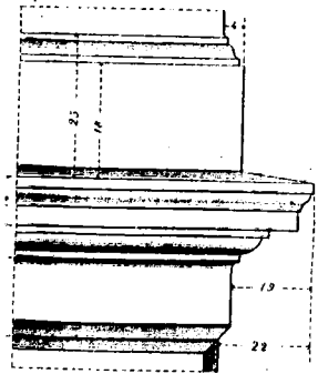
Fig. 9ª Cornicione della facciata, e capitello dello paraste.
