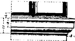
Fig. 6ª Cimasa del parapetto del 1° piano.
