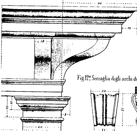
Fig. 9ª Cornicione della facciata, e capitello dello paraste.
