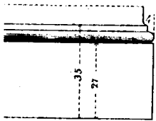
Fig. 3ª Particolari dello zoccolo della facciata.
