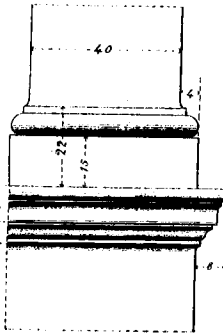
Fig. 9ª Cornicione della facciata, e capitello dello paraste.
