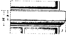
Fig. 6ª Cimasa del parapetto del 1° piano.
